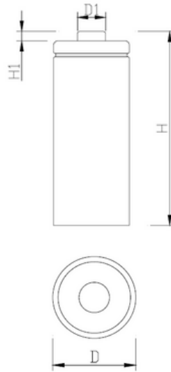
Dimensions(GB)
